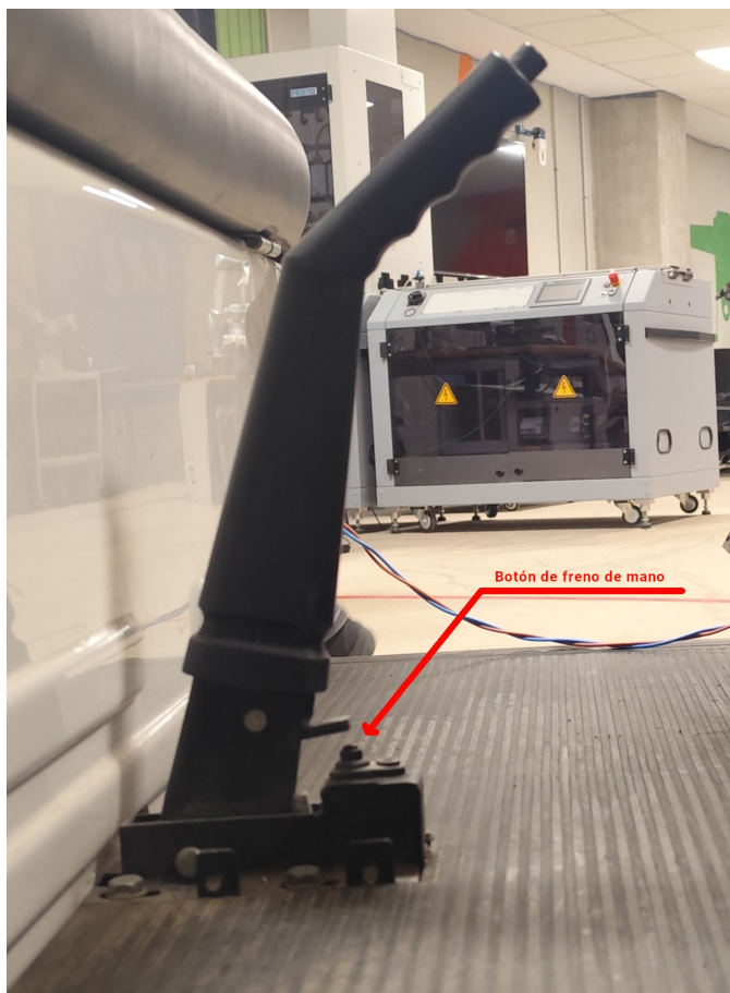
Activado (Arriba) - Interruptor Cerrado
